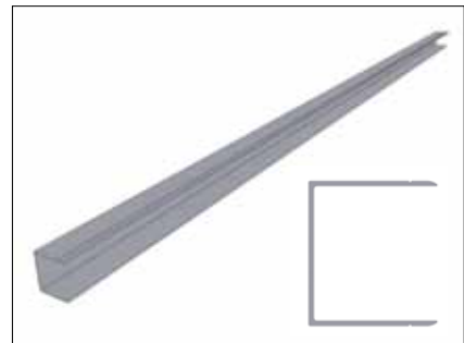
П-профиль панелей притолоки L=2855 - 1шт.
