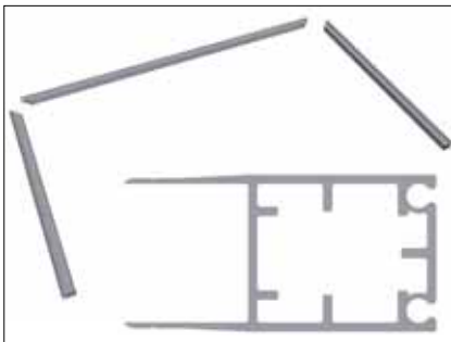
Профиль нижний несущий окан- товки проема L=2290x45(1)° - 2шт. L=3179x45(2)° - 1шт.
